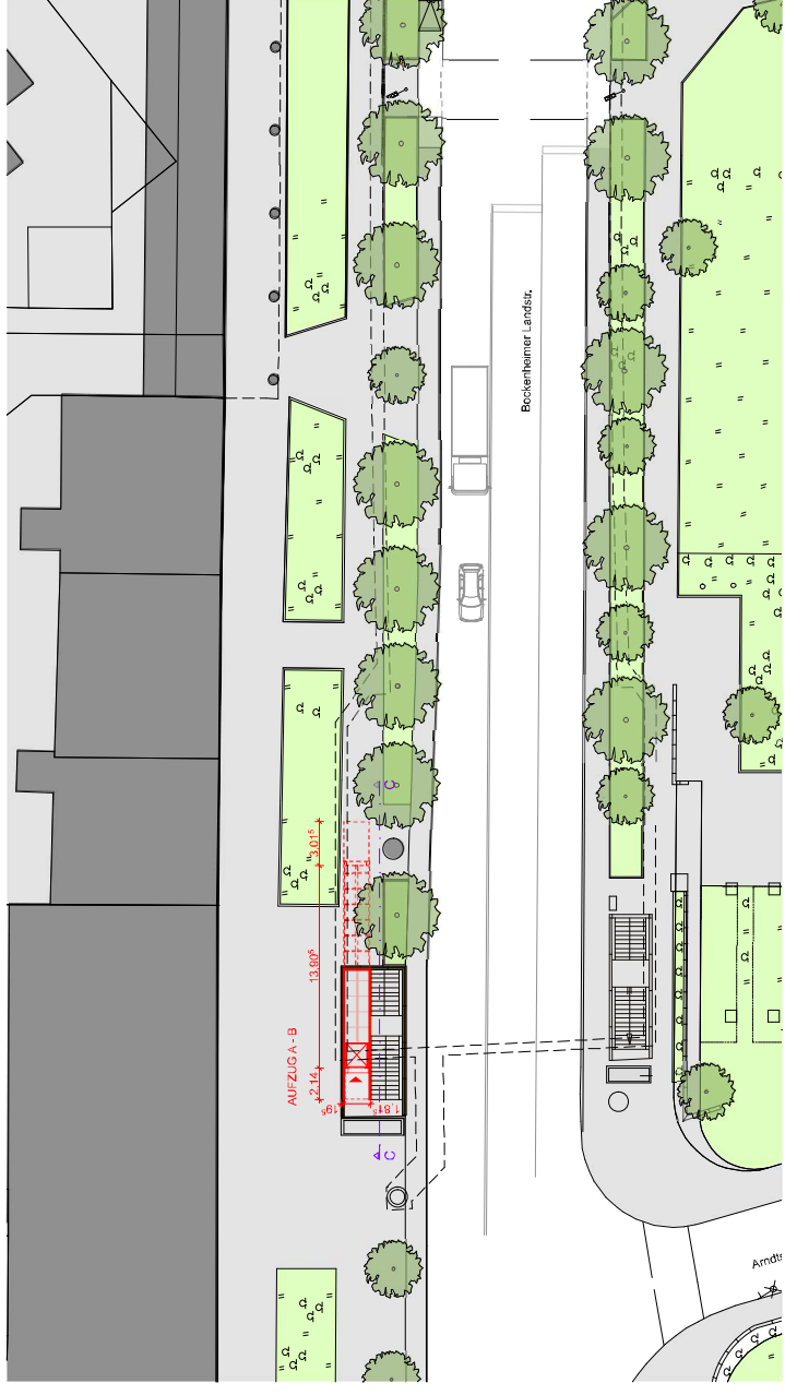
Ausschnitt A - Ebene M 1:200
